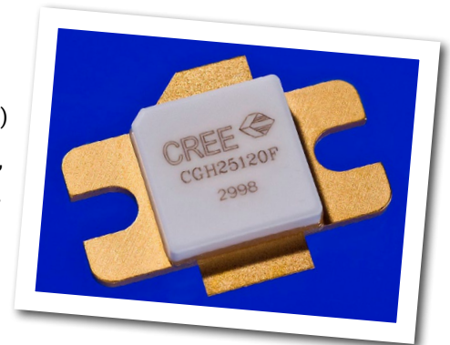
Package Type: 440162 PN: CGH25120F
